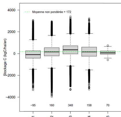
Figure 4-18. Variation moyenne annuelle absolue du stock de C (kgC/ha/an) dans l'horizon 0-30 cm des prairies permanentes productives (tous modes d'exploitation confondus) en fonction de la texture du sol
