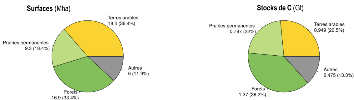
Figure 2-11. Surfaces et stocks totaux de carbone par grand type d'usage des terres, estimés d'après le RMQS. Les surfaces en terres arables incluent les surfaces en prairies temporaires (< 6 ans) et prairies artificielles.
