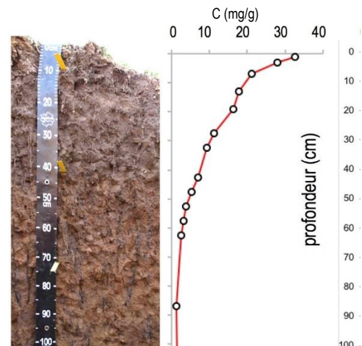
Figure 1-2. Profil de sol de prairie et distribution verticale du carbone organique de ce sol
