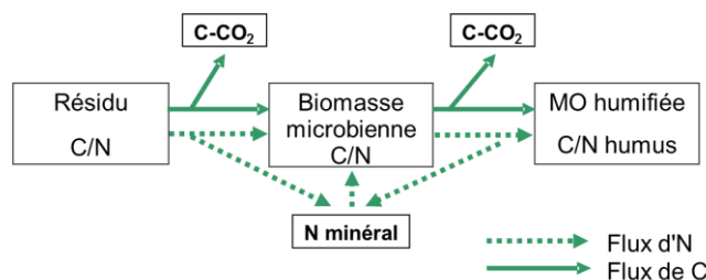
Figure 2-8. Représentation simplifiée des interactions C-N dans le modèle STICS
