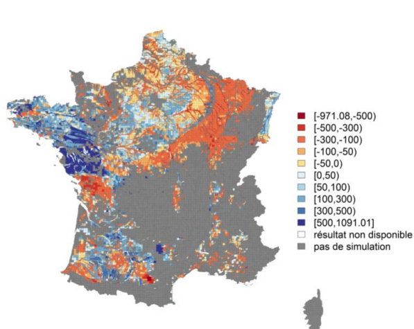
Figure 4-3. Stockage de carbone annuel absolu (kgC/ha/an) sur l'horizon 0-30 cm pour les systèmes de grandes cultures et prairies temporaires simulés sur 30 ans avec STICS
