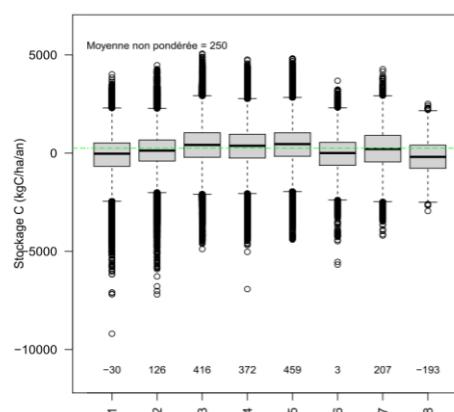
Figure 4-19. Variation moyenne annuelle absolue du stock de C (kgC/ha/an) dans l'horizon 0-30 cm des prairies permanentes productives (tous modes d'exploitation confondus) en fonction du climat
